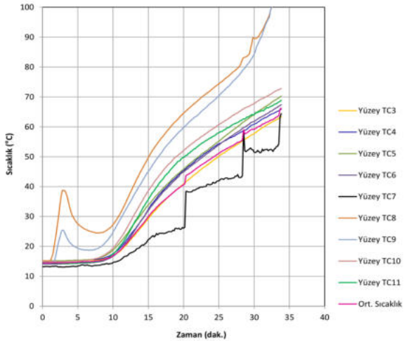
Şekil B2: Kapi No.1'nin yüzey sıcaklıkları (TC3 – TC11 ve Ort. sıcaklık)
