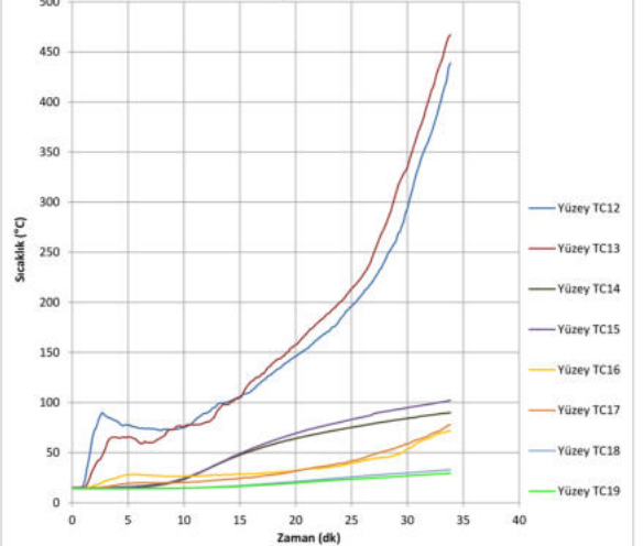
Şekil B3: Kapi No.1'nin yüzey sıcaklıkları (TC12 – TC19).
