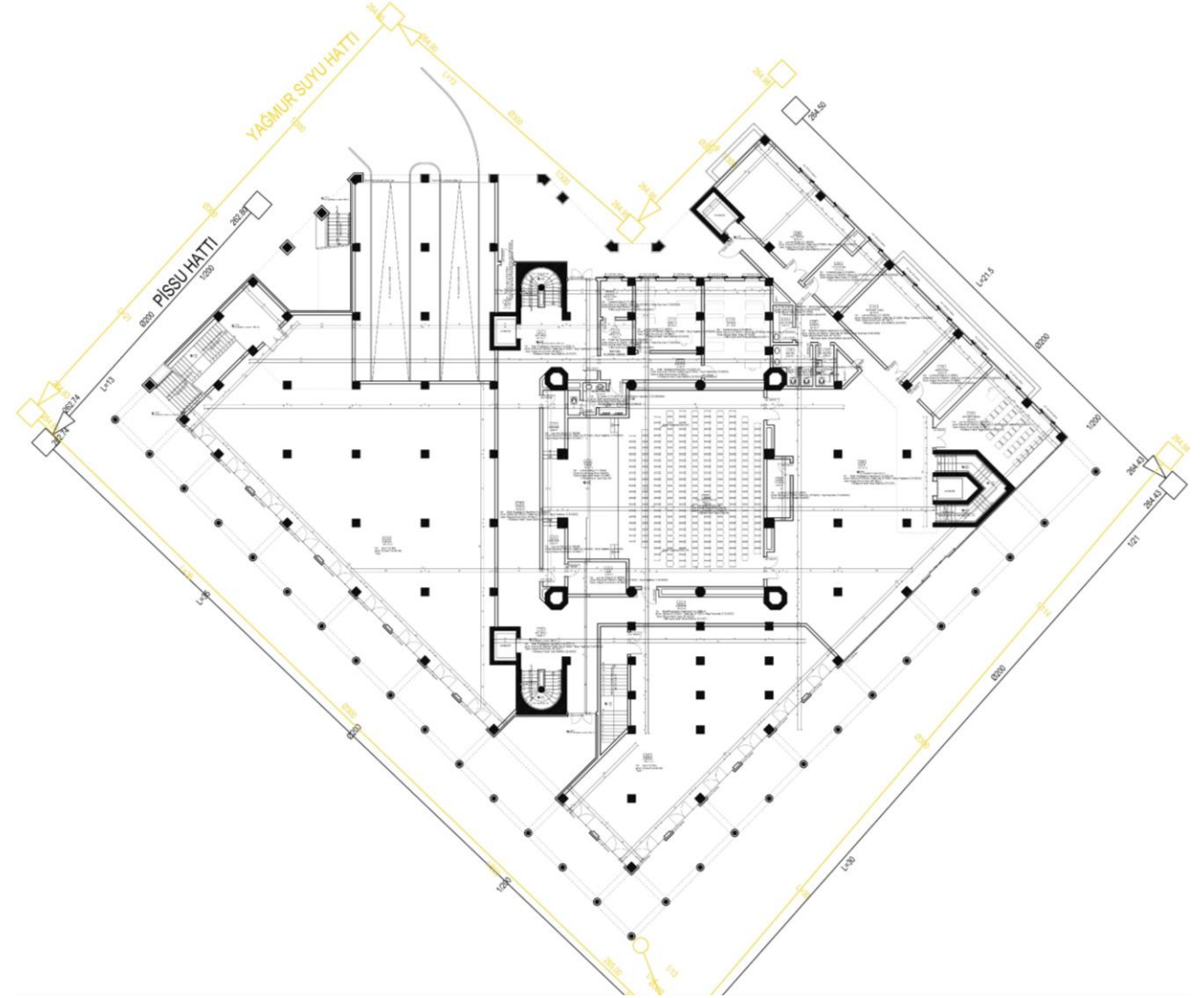
ZEMİN KAT PLANI
