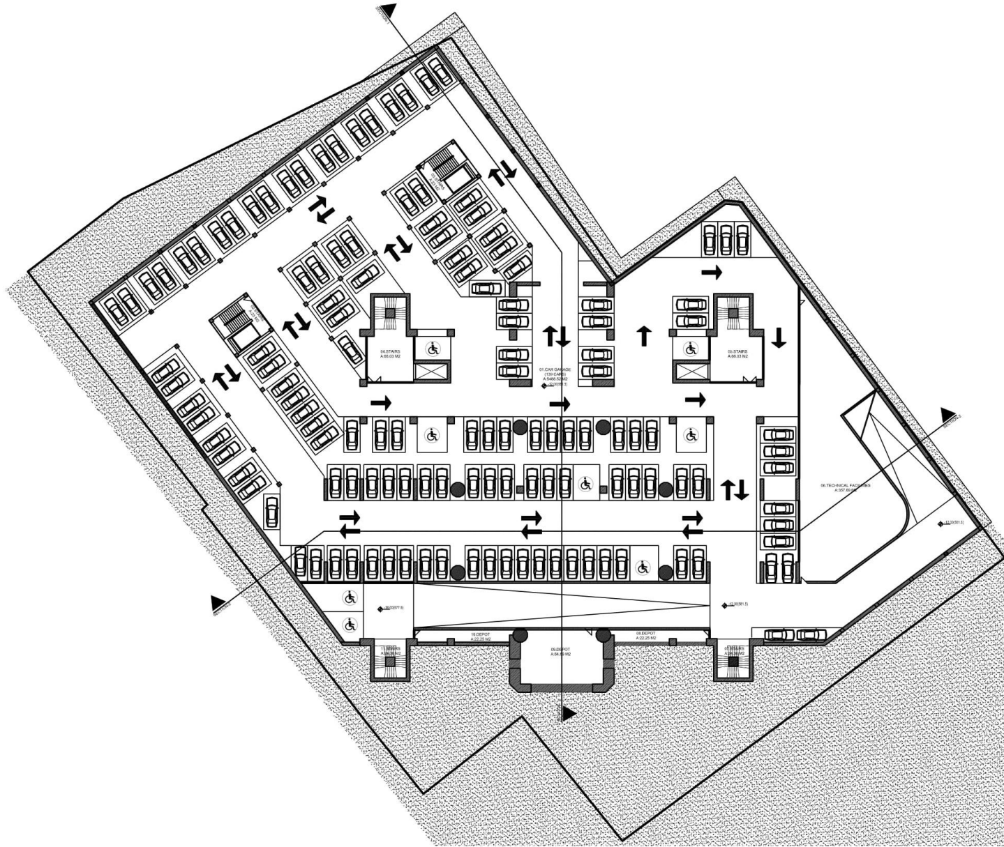
3-4-5-6. BODRUM KAT PLANI
