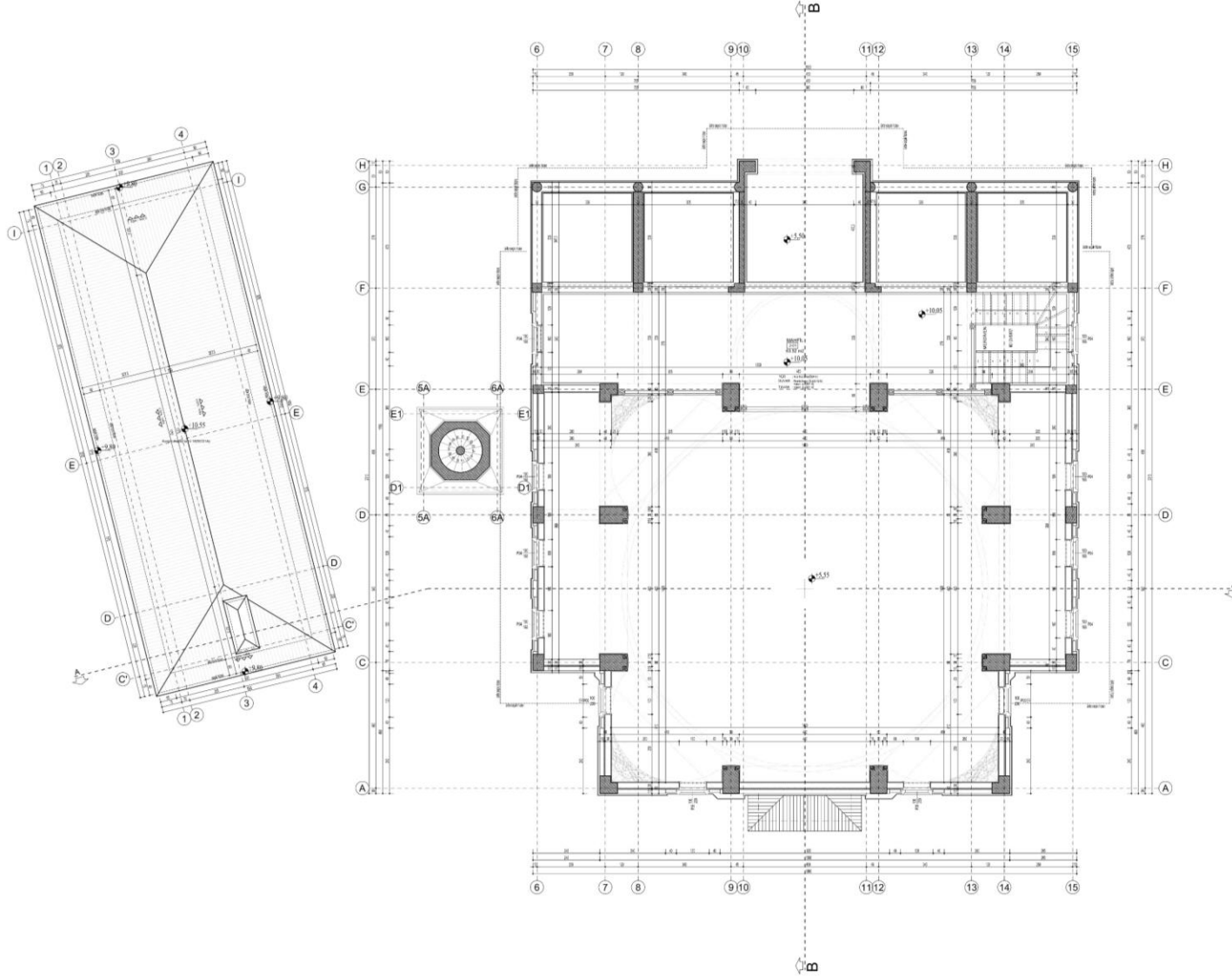
MAHFİL KATI PLANI
