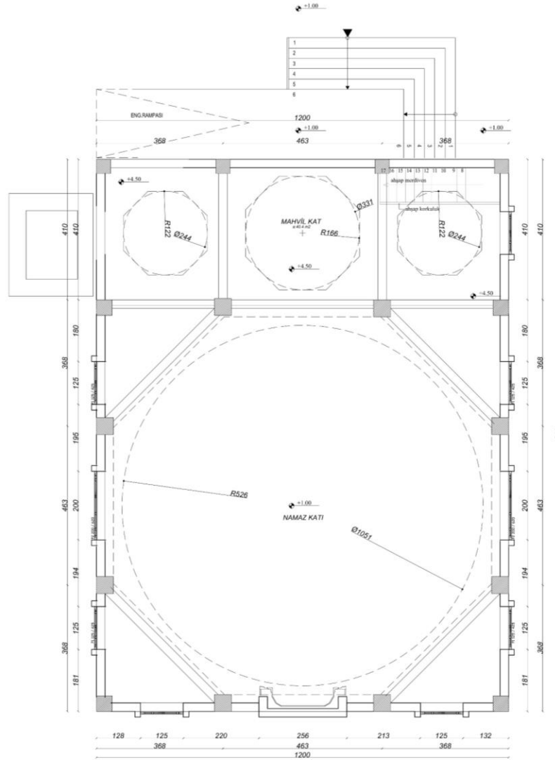
MAHVİL KAT PLANI
